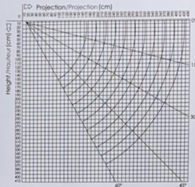
Wall covering diagram - Surface de couverture au mur
