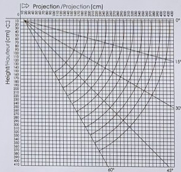
Ceiling covering diagram - Surface de couverture au plafond
