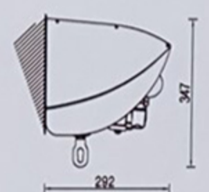
Installation with a hood Installation avec auvent
